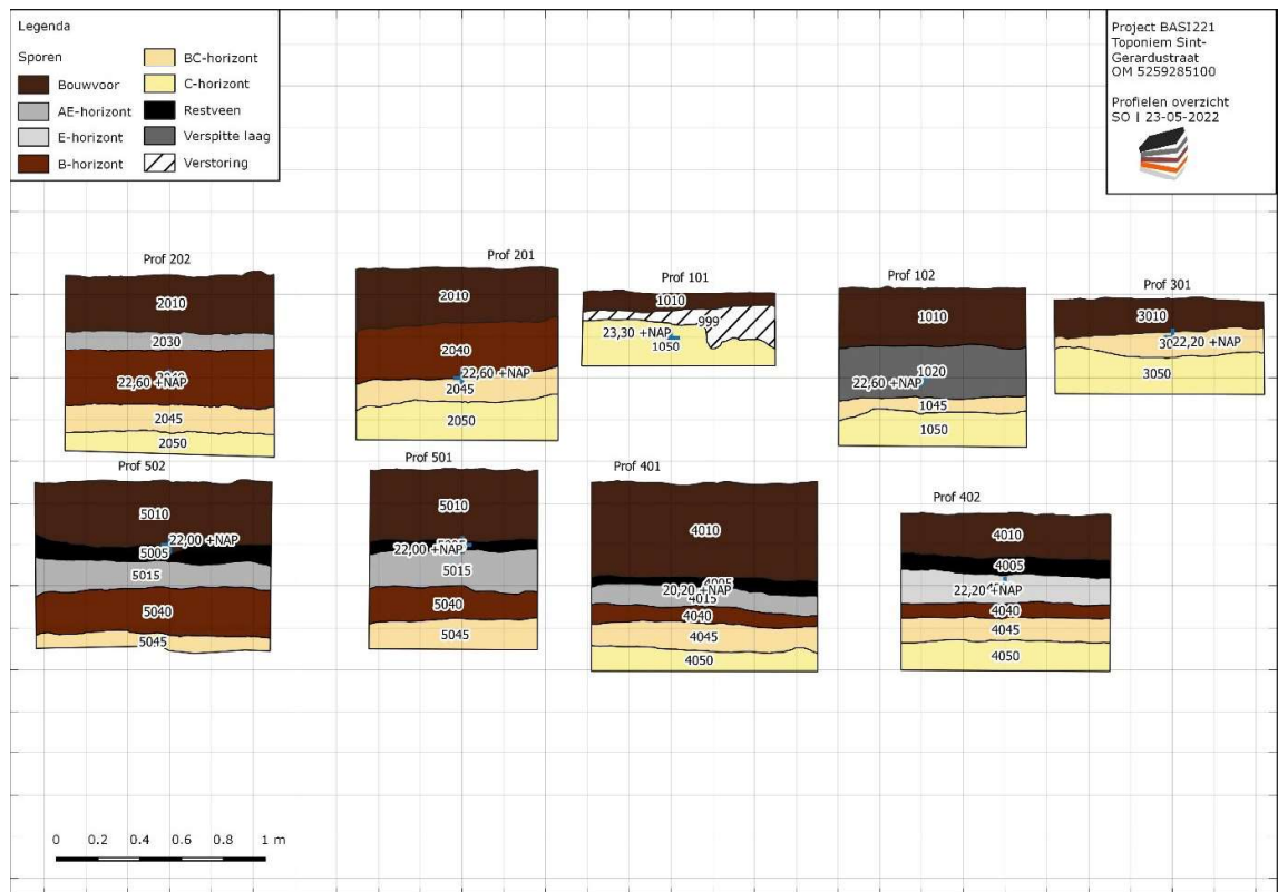
Afbeelding 3. Schematisch overzicht van de profielen.
