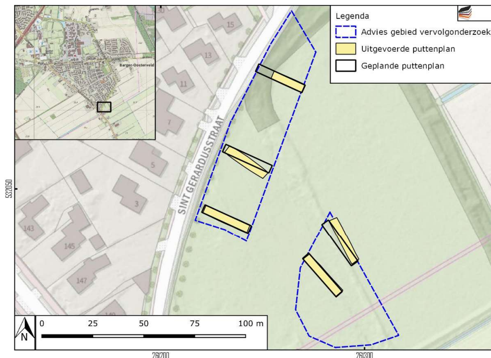
Afbeelding 2. Geplande puttenplan over het uitgevoerde puttenplan.
